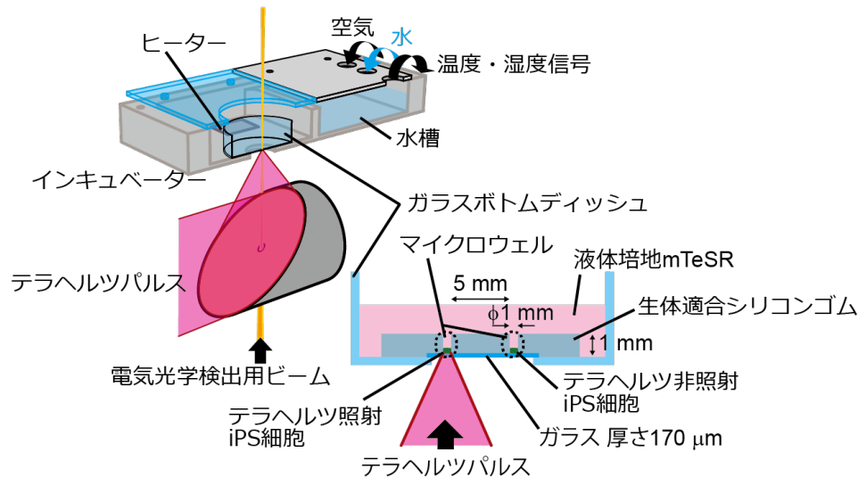
図 iPS 細胞を培養しながら、テラヘルツパルス照射を可能とする装置 直径 1mm のマイクロウェルにて iPS 細胞を培養することで、均一にテラヘルツパルス を照射することが可能となった。
