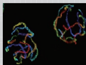
図2：私たちが開発した定量的イメージ解析プログラムの一例。顕微鏡画像を元に、解析プログラムが自動でヒト幹細胞核を検出し、DNAやヒストン修飾濃度の分布を核膜周辺から核の内部に向けて定量化する。
