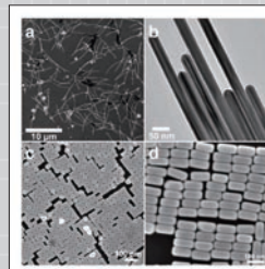
金ナノ粒子の形態制御合成 (aとb: ナノワイヤー、c: ナノ立方体、d: 四角立方体)
