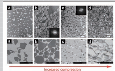
Langmuir-Blodgett法を用いて形成したナノスケール構築要素の2次元 (2D) 的な集合体 (上: BaCrO 3 ナノロッド、下: グラフェン酸化物ナノシート)
