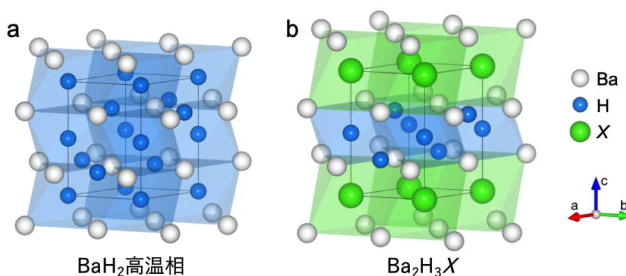
図2. a) これまでで最高の \text{H}^- イオン伝導度を示す \text{BaH}_2 高温相の結晶構造。ただし、 450^\circ\text{C} 以上でのみ安定に存在。b) 本研究で着目した層状アニオン秩序をもつ \text{Ba}_2\text{H}_3\text{X} ( \text{X} = \text{Cl}, \text{Br}, \text{I} )。BaH2高温相
