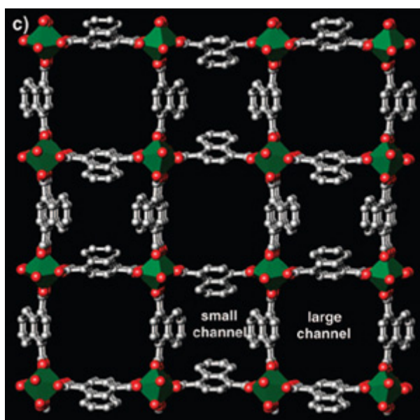
図2 ナノ孔物質 \text{Al(OH)(1,4-NDC)} の結晶構造
