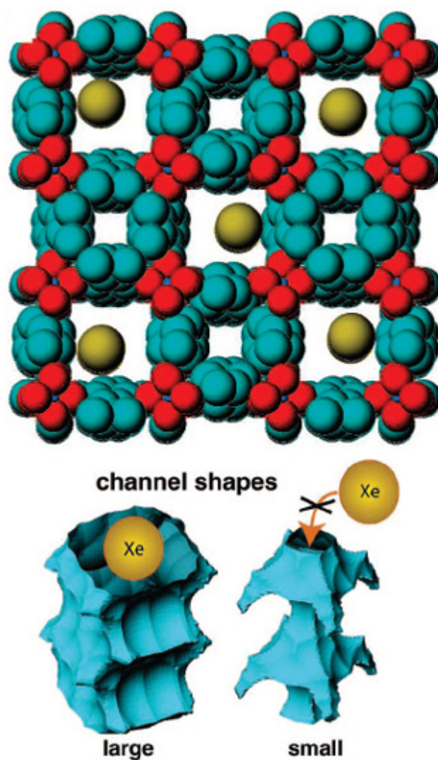
図3 (上) 固体 NMR 測定の結果から得られたキセノンガス分子吸着のモデル図
